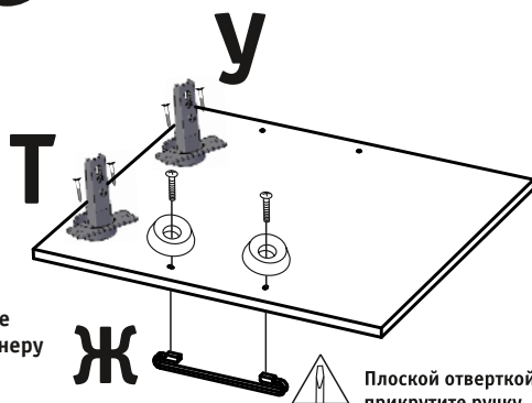
Рис. 1. Установка ручки и петель.
