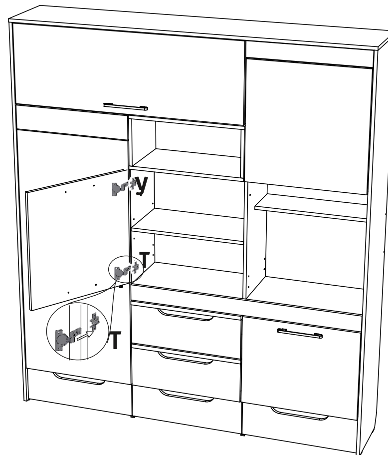
Рис. 2. Схема установки маркерной доски
