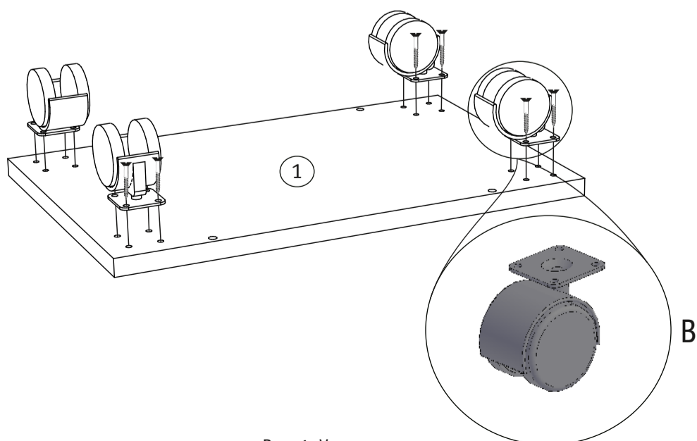
Рис. 1. Установка опор.
