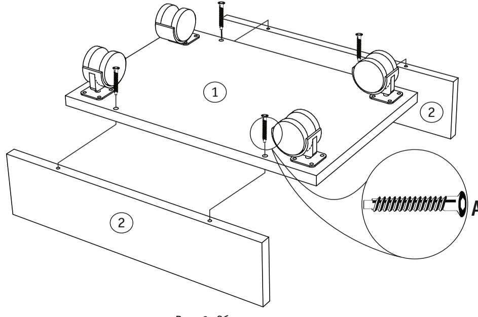
Рис. 2. Сборка каркаса.
