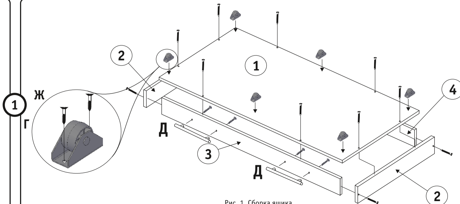
Рис. 1. Сборка ящика.
