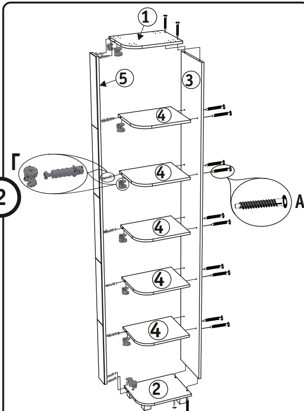
Рис. 2. Сборка каркаса.
