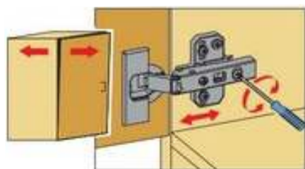
Рис. 5. Регулировка фасада.
