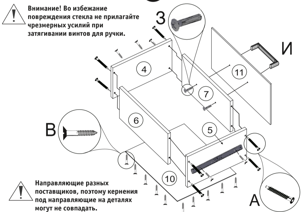
Рис. 5. Сборка ящика.
