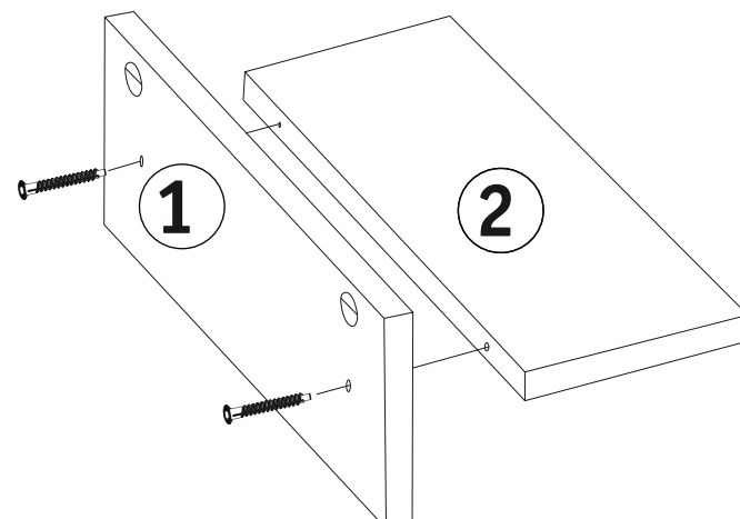
Рис. 1.2 Сборка полки (Сенатор 9, Кристалл 9).
