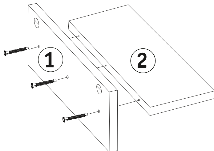
Рис. 1.1 Сборка полки (Сенатор 8, Кристалл 9, София 11, София 12, Оливия 11).
